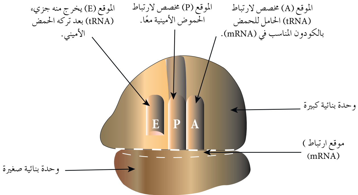
الشكل (٤ - ٤٩): تركيب الرايوسوم.
