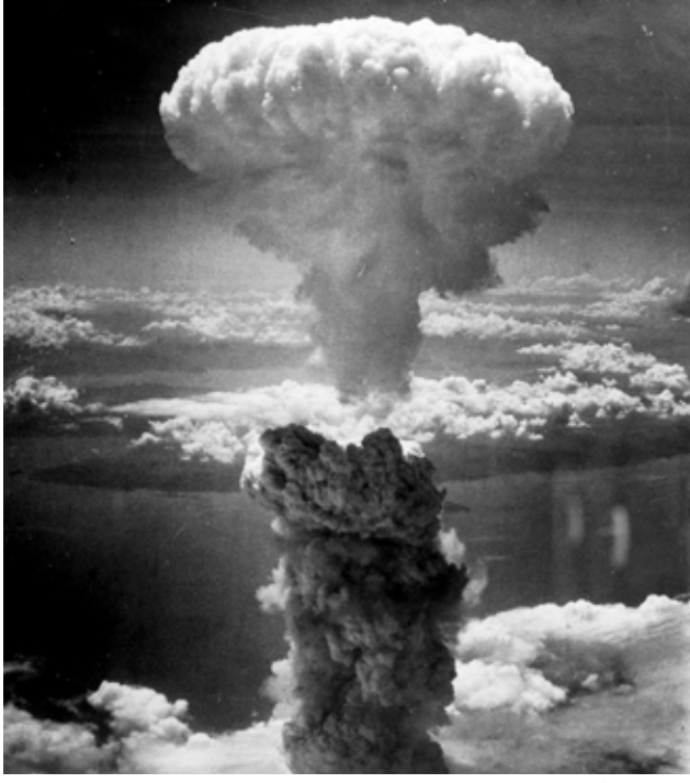
الشَّكْلُ (٣١-٤) السَّحَابَةُ الناتجةُ عَنْ إسْقَاطِ القنبلةِ النوَوِيَّةِ على مَدِينَةِ (ناجازاكي) في اليابان عامَ (١٩٤٥)
