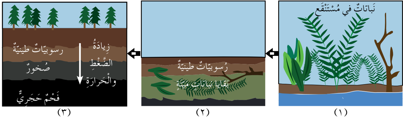
الشكل (٥-٩): مراحل تكوين الفحم الحجريّ.
