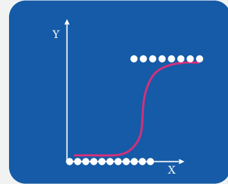
الشكل (2-6): مثال على الانحدار اللوجستي
