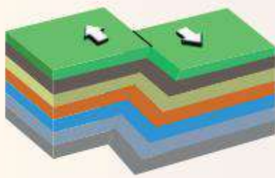
صدع جانبي
