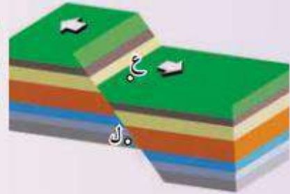
صدع عادي
