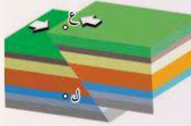
صدع عكسي
