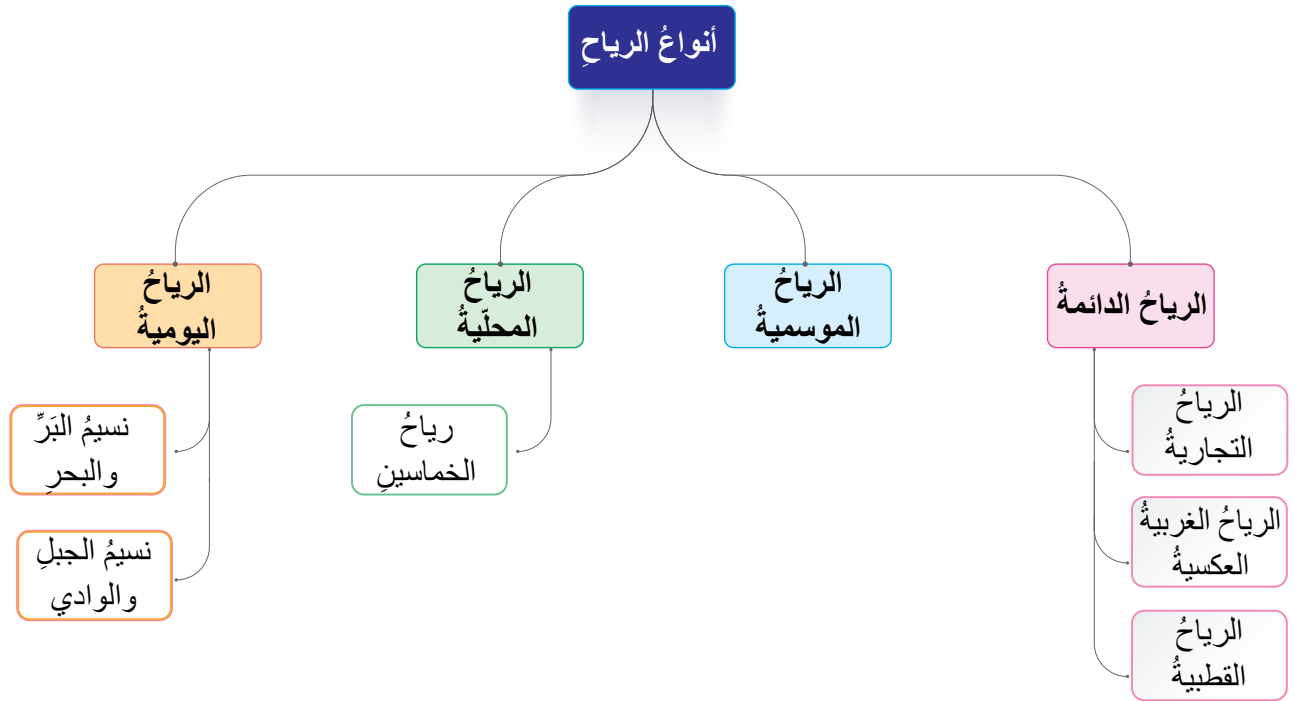
الشكل (5): أنواع الرياح.
