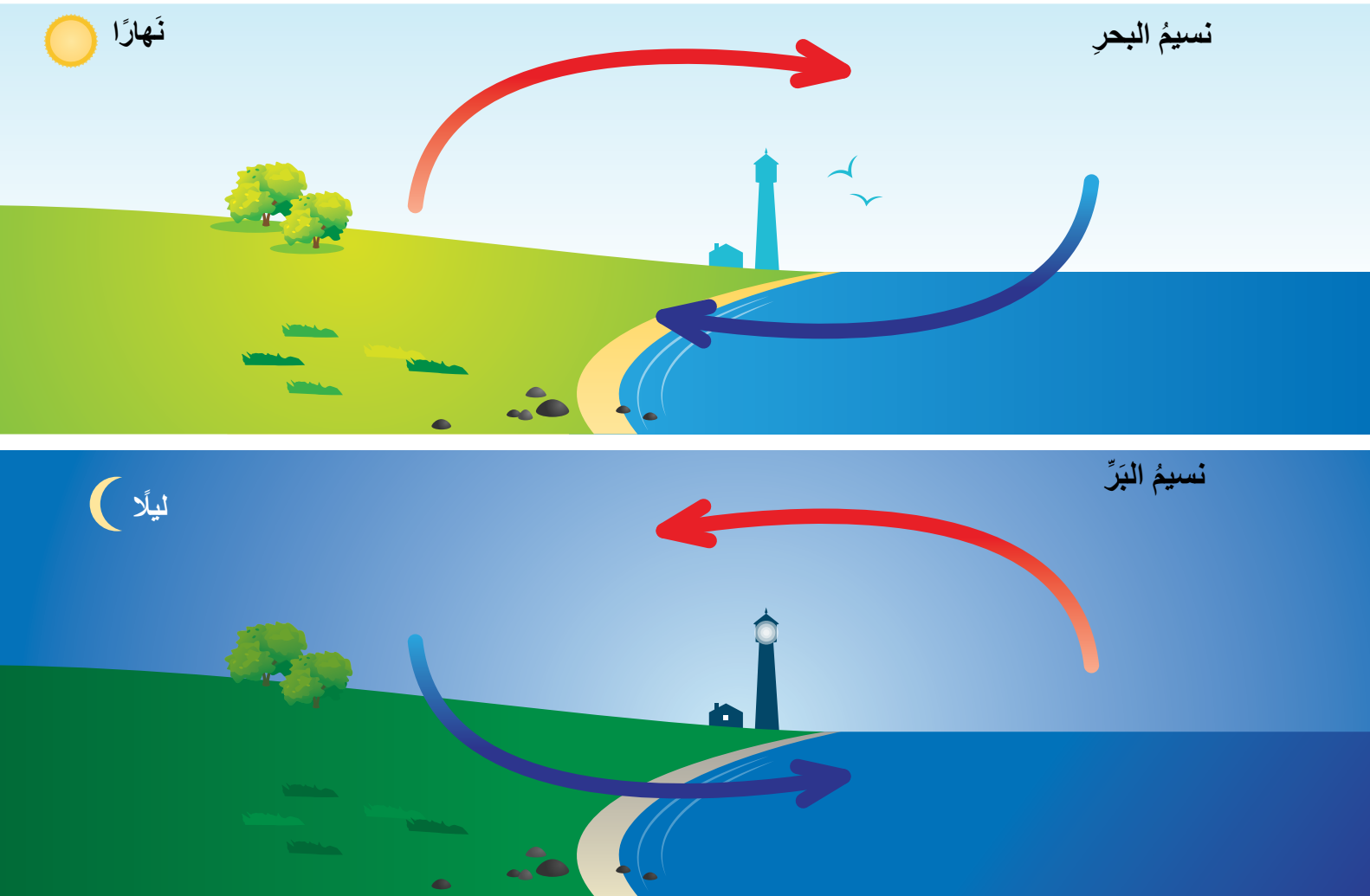
الشكل (6): آلية حدوثِ نسيمِ البرِّ ونسيمِ البحرِ.
