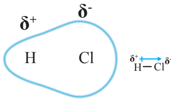
الشكل (29): قطبيّة الرابطة في جزيء \text{HCl} .
