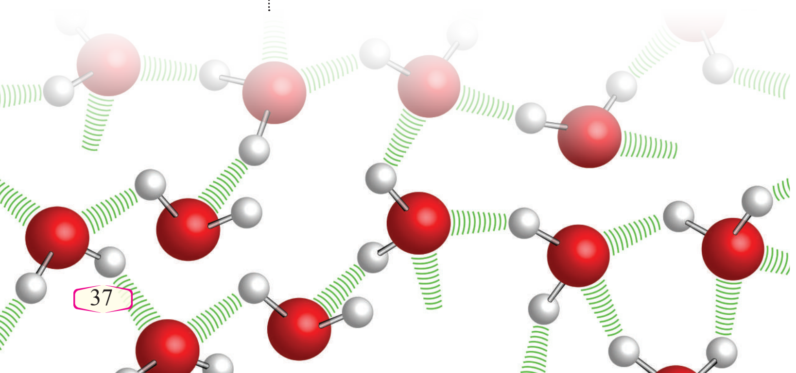
الشكل (35): الروابط الهيدروجينية بين جزيئات الماء.
