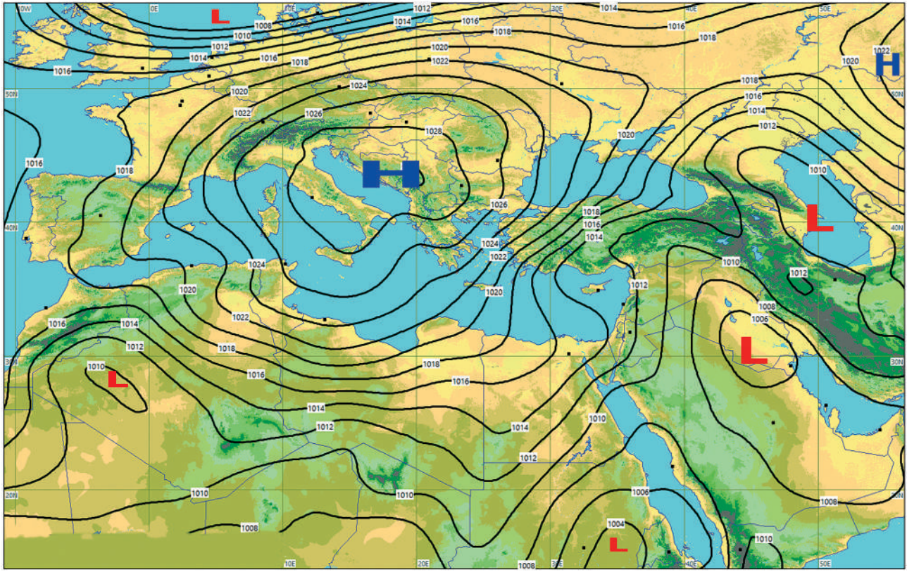
الشكل (6): خريطة طقس سطحية تبين أنظمة الضغط الجوي.
