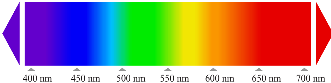
الشكل (6): الضوء المرئي.
