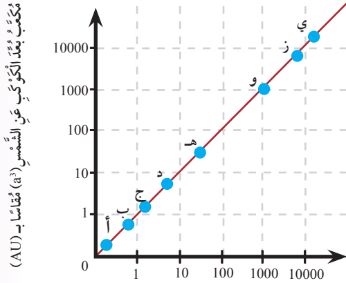
مربع زمن دوران الكوكب حول الشمس ( P^2 ) بوحدة (earth years)
