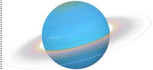
الشكل (11): كوكب أورانوس.
