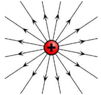
شحنة نقطية موجبة
