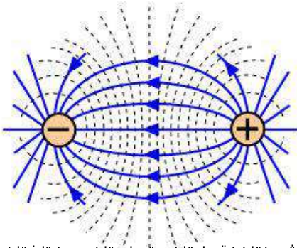
شحنتان نقطيتان متجاورتان ومختلفتان نوعاً ومتساويتان مقداراً
