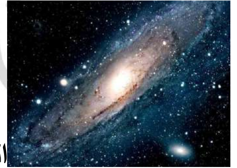
الكواكب والنجوم
