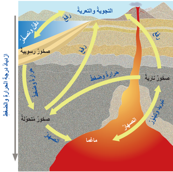
الشكل (1): دورة الصخور في الطبيعة. أأخذ: ما المرحلة التي يجب أن تمر بها الصخور جميعاً لتُشكّل الصخور النارية؟
