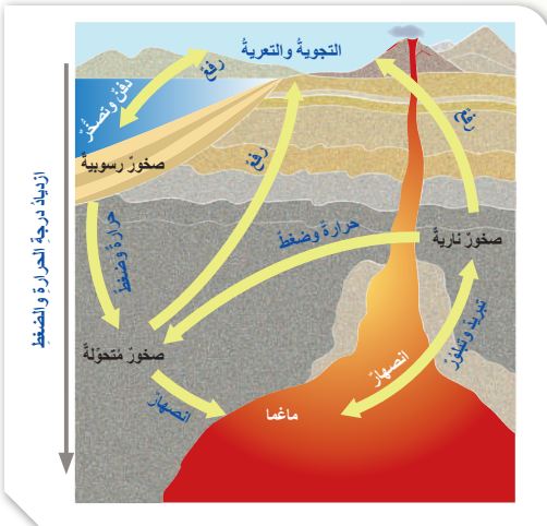
الشكل (1): دورة الصخور في الطبيعة. أُنظر الشكل (1) الذي يُمثّل هذه الدورة.
