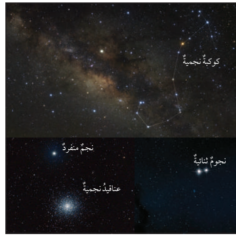
الشكل (4): الأشكال المختلفة للنجوم في السماء. أصف الشكل الذي تظهر به العناقيد النجمية.
