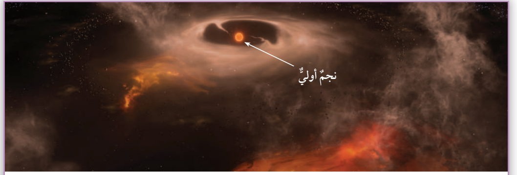
الشكل (10): ولادة النجم الأولي من السديم.
