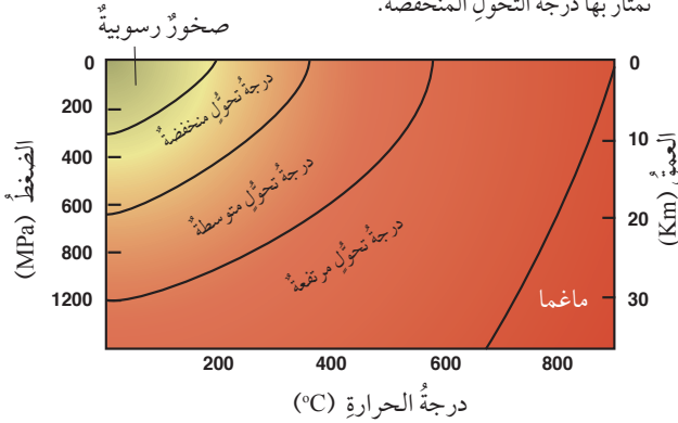
الشكل (22): درجات التحول في الصخور المُتحوّلة. أستخدم: أي الصخور تتكوّن في أعلى درجة تحول؟
