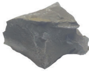
الشكل (25): الصخر الزيتي الذي يتوافر بكميات اقتصادية في وسط الأردن وشماله.
