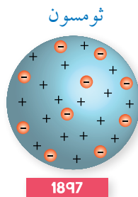
الشكل (1): بعض النماذج الذريّة.
