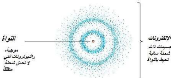
الشكل (11): التركيب العام للذرة
