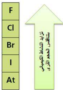
الشكل (16): تزايد نشاط عناصر المجموعة 7A
